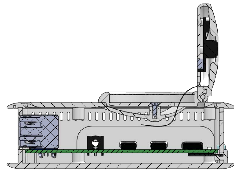
SEZIONE A-A
